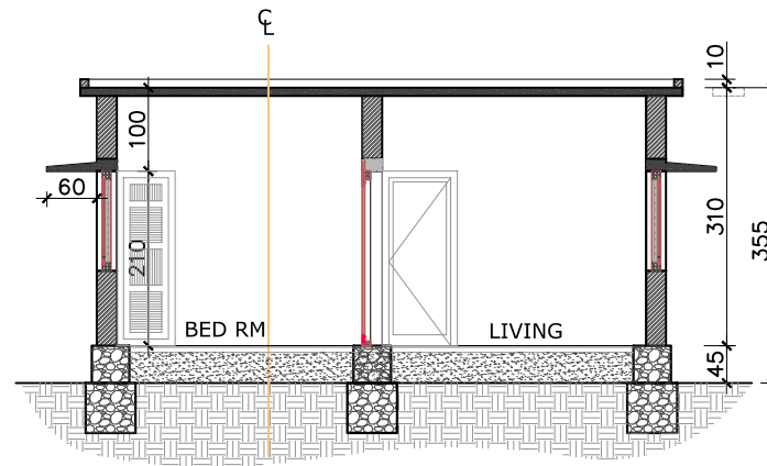
3 SECTION-A
